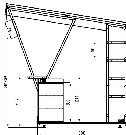
SEZIONE A-A
